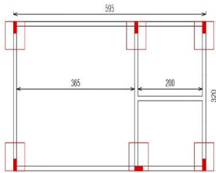
PLANTA BAIXA - PILARES E BLOCOS ESC. 1/50
