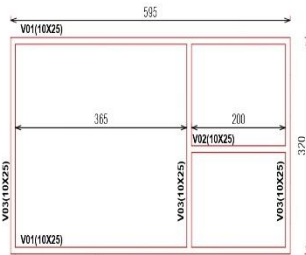
PLANTA BAIXA - VIGA TRAVAMENTO 01 NÍVEL +2,55 ESC. 1/50
