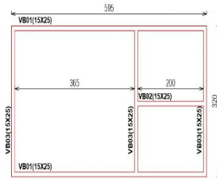
PLANTA BAIXA - VIGA BALDRAME NÍVEL +0,00 ESC. 1/50
