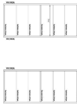
PLANTA BAIXA - VIGA TRAVAMENTO 01 E 02 ESC. 1/50
