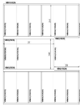
PLANTA BAIXA - VIGA BALDRAME ESC. 1/50
