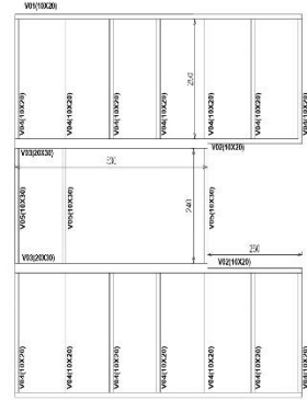
PLANTA BAIXA - VIGA TRAVAMENTO 03 ESC. 1/50
